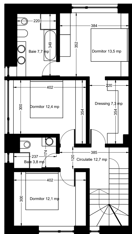
Plan etaj
