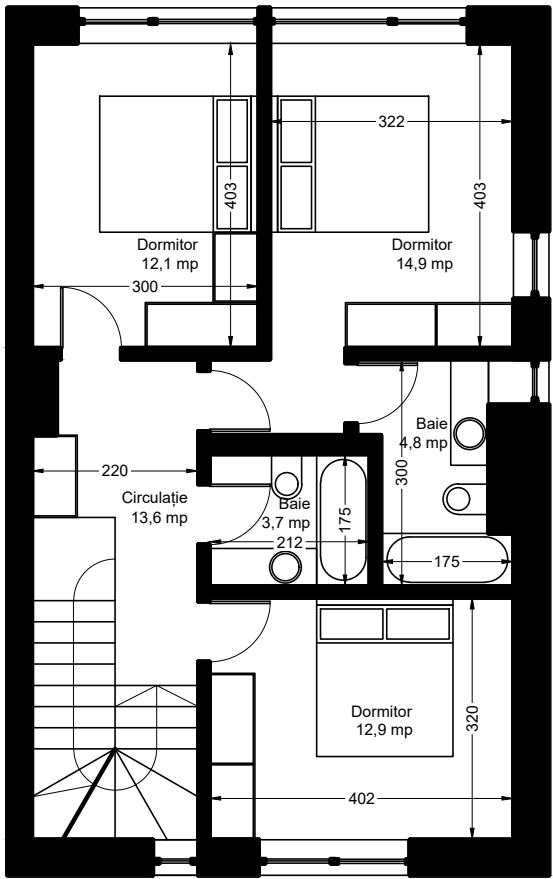
Plan etaj
