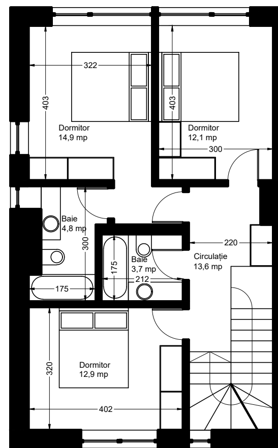
Plan etaj
