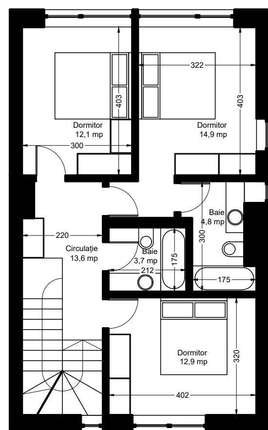
Plan etaj
