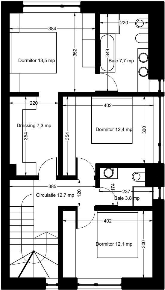
Plan etaj
