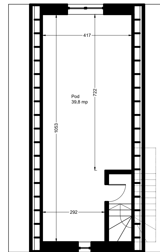
Plan mansardă neamenajată
