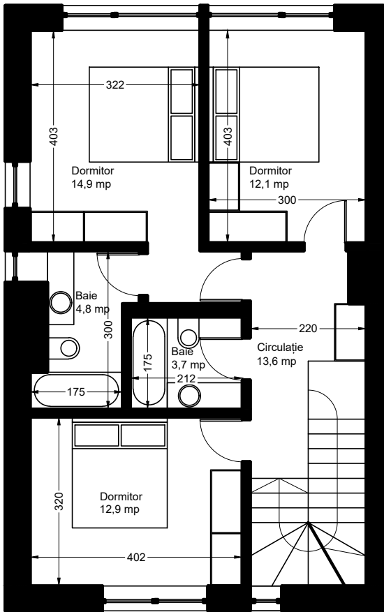
Plan etaj
