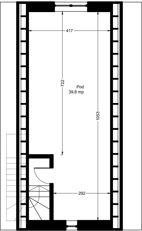
Plan mansardă neamenajată
